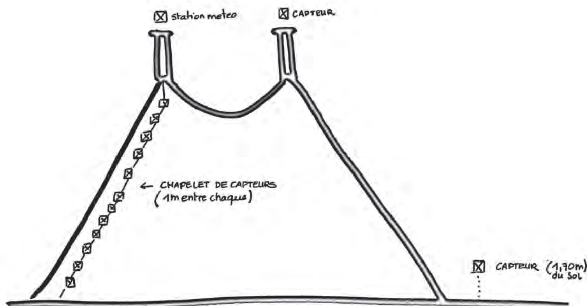
Dessin du procédé mis en place pour analyser les températures des chapiteaux. © Louis Cormerais
